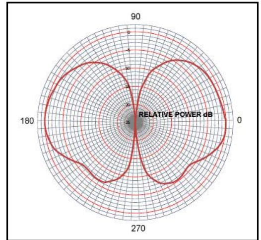
AS-390 (UHF) – ELEVATION
