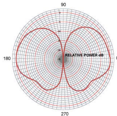
AS-390 (UHF) – ELEVATION
