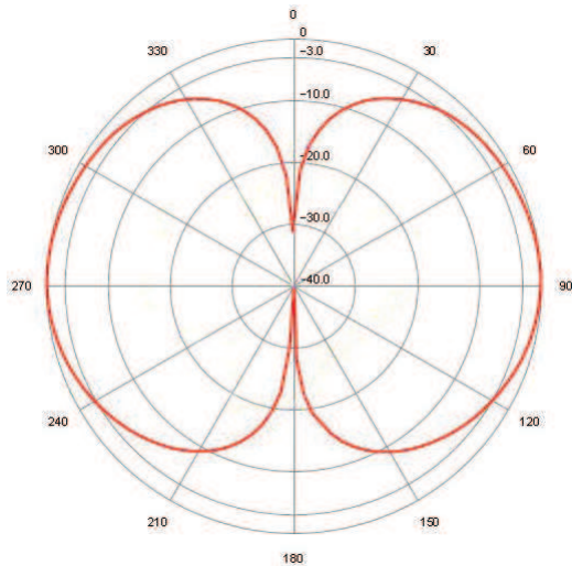
UHF E-PLANE
