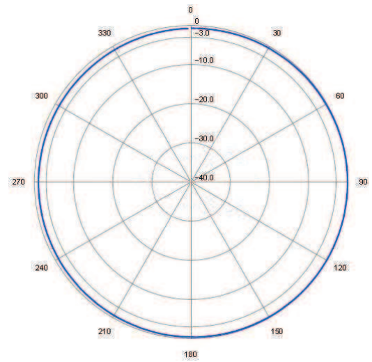
VHF E-PLANE
