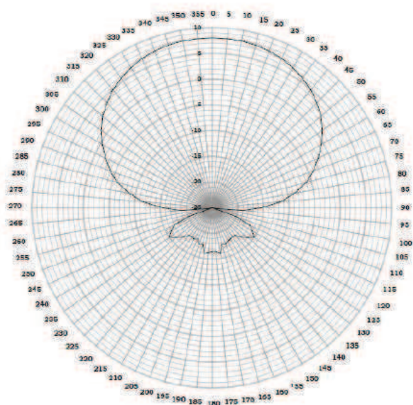
LPD-7 H-PLANE
