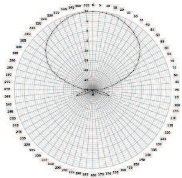
LPD-12 H-PLANE
