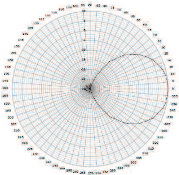
LPD-12 E-PLANE
